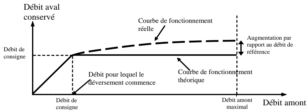
Figure 104 : Principe de fonctionnement hydraulique du déversoir d'orage
