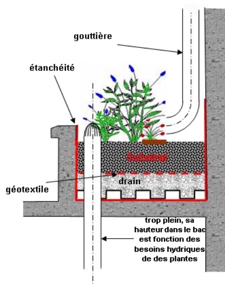
Figure 41 : Coupe de principe et illustration montrant une jardinière sur dalle dans laquelle se jette la gouttière d'un immeuble
