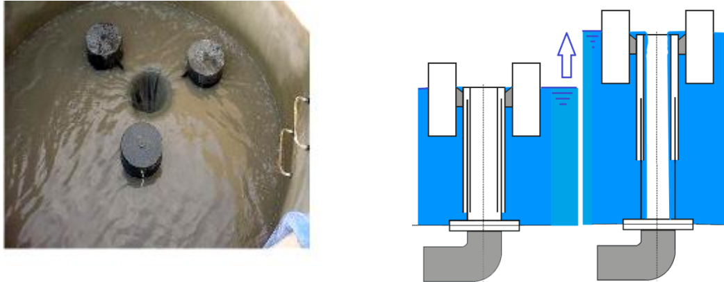
Figure 131 : Déversoir flottant (ISMA)
